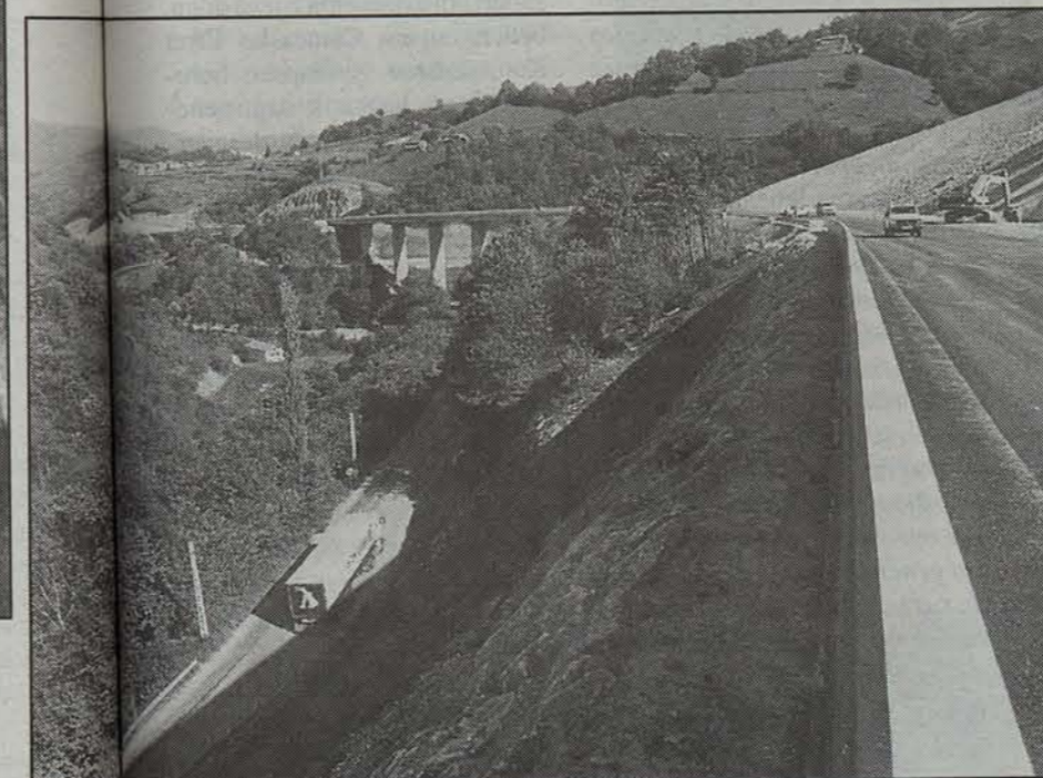
Belateko tunelaren irteera. Eskuinean, Belateko eta Almandozko tunelaren bitarteko zatia, eta Almandozko tunelaren irteera. Ezkerrean, lanak Almandozko tunelaren barruan eta hemen behean, Almandozko tunelaren zati eta Marin erreka zubia. Beherago, Almandozko lurren mugimendua. OSKAR MONTERO
